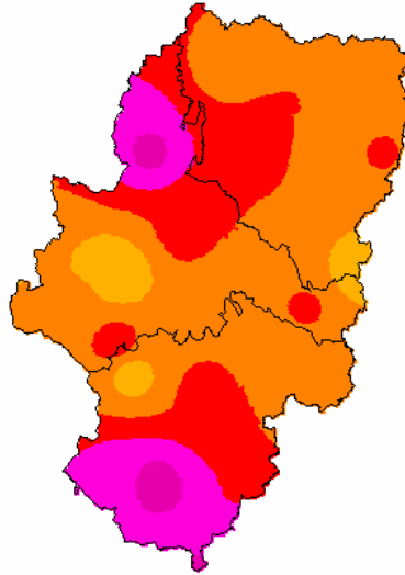
SPI12 (junio de 2020)
