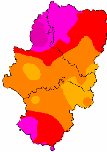
SPI6 (junio de 2020)
