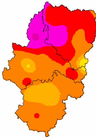
SPI24 (junio de 2020)
