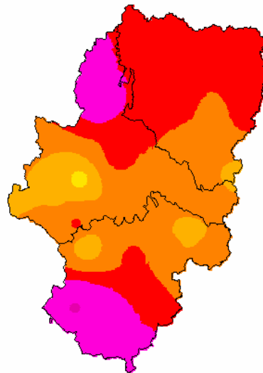
SPI3 (junio de 2020)
