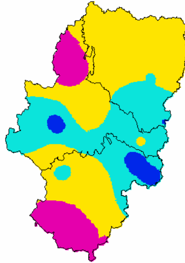
¿ RESPECTO NORMAL PRECP AÑO AGRICOLA (junio de 2020)
