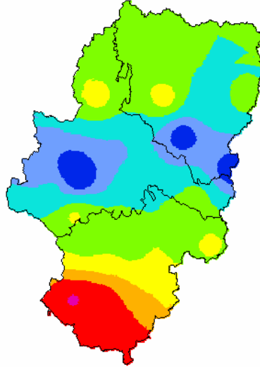
ANOMALIA DE LA PRECIPITACION (%) (junio de 2020)
