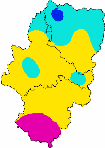
ANOMALIA TEMPERATURA MEDIA (junio de 2020)
