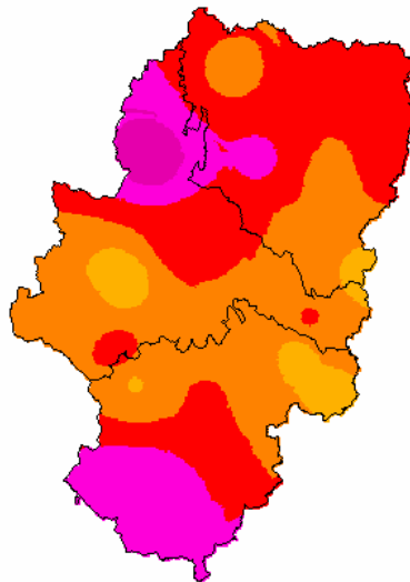
SPIAÑOAGRICOLA(10 MESES) (junio de 2020)
